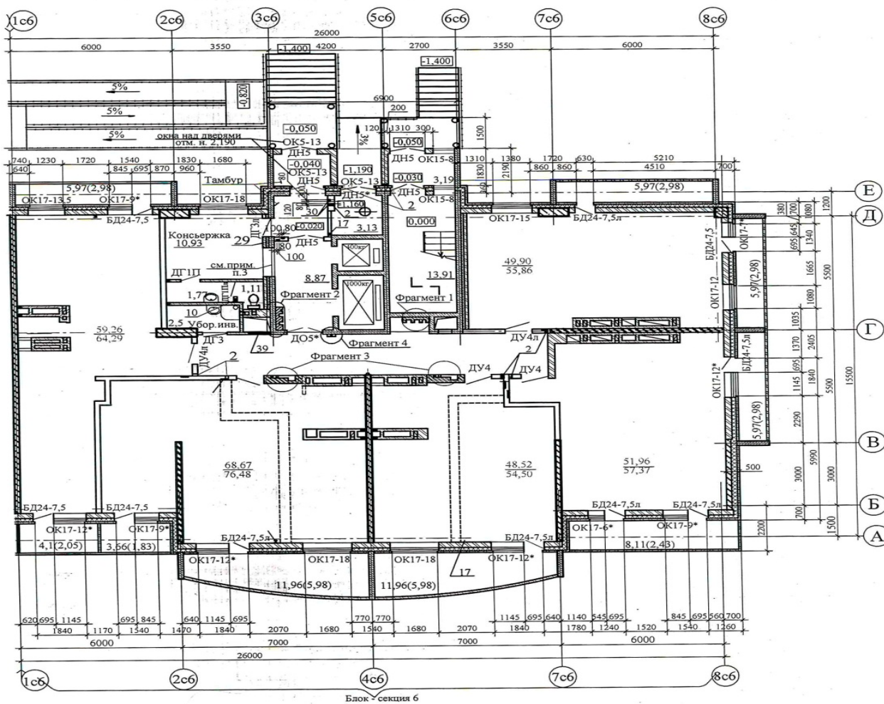
План б б/с, 1 этаж
